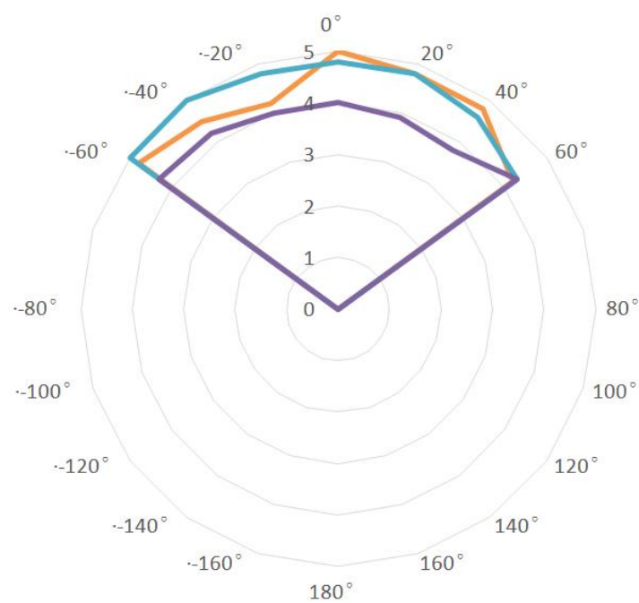
图 10 探测范围示意图(挂壁高度1.5米)
