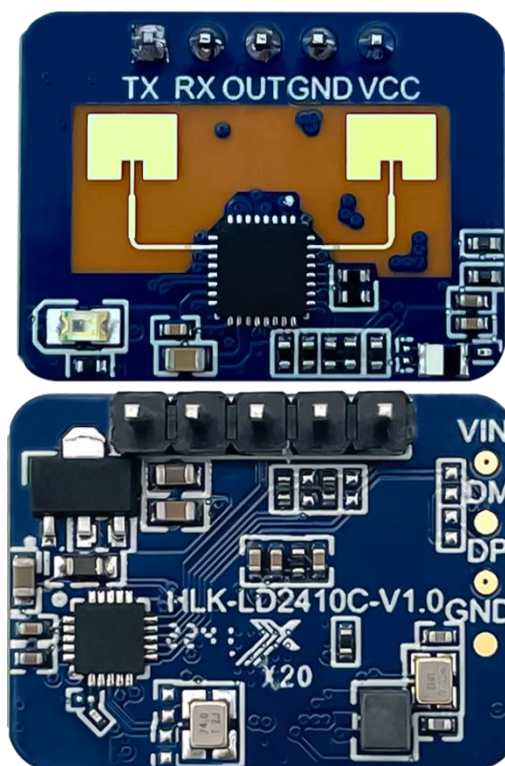
图 4 模块实物图
