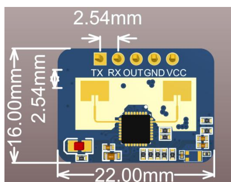
图 5 模块尺寸图
